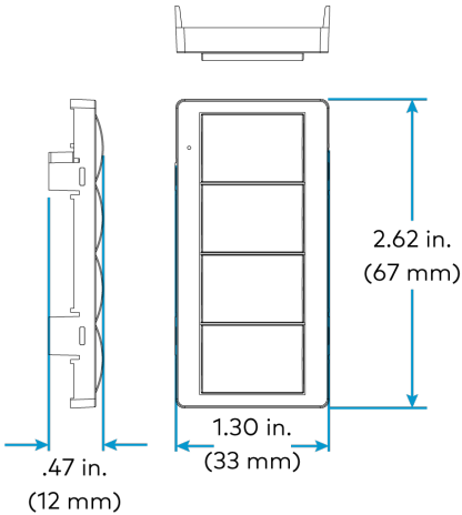
ZUMLINK-BTN4 (BLANK shown)
