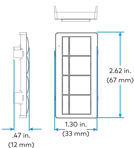
ZUMLINK-BTN8 (BLANK shown)
