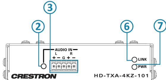
HD-TXA-4KZ-101 Front Panel
