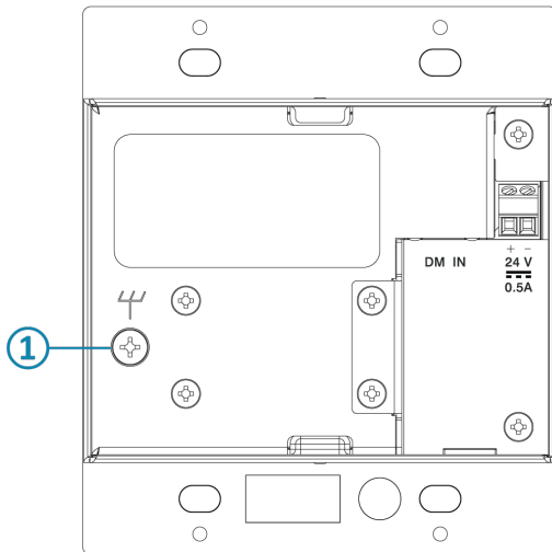
HD-RXU-4KZ-101-2G, Rear
