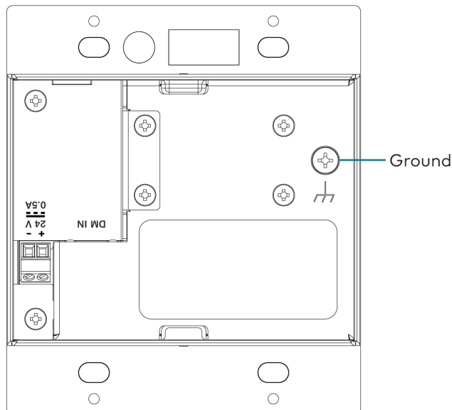
HD-RXU-4KZ-101-2G Rear
