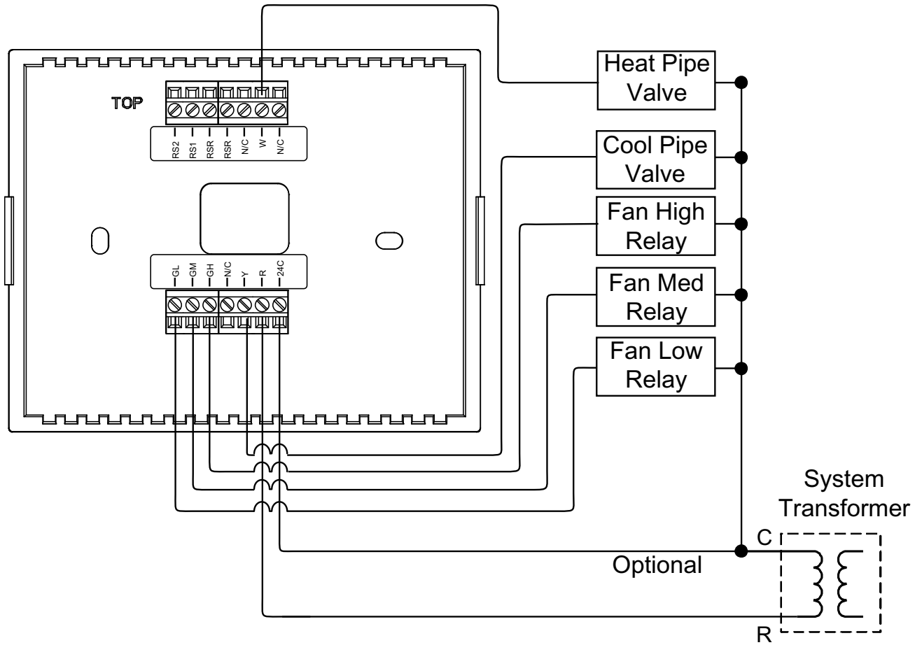
CHV-TSTATEX-FCU Wiring Diagram
